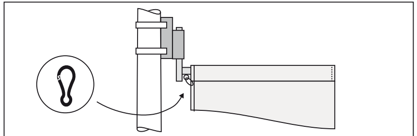
Vormontage vom Basisteil und vom Kordelhalter (optional) am Kandelaber
