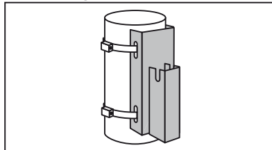
Vormontage vom Basisteil und vom Kordelhalter (optional) am Kandelaber
